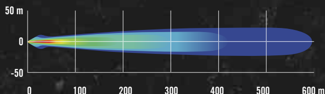
XL Sport-strålkastare
