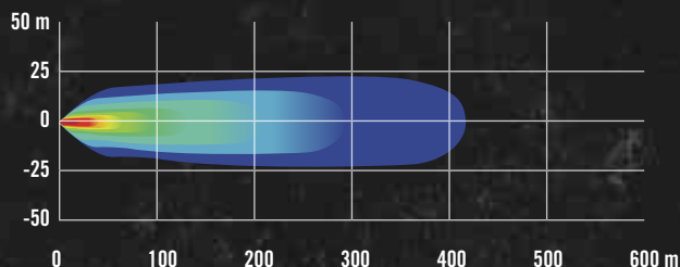
XL80 – kombinationsläge
